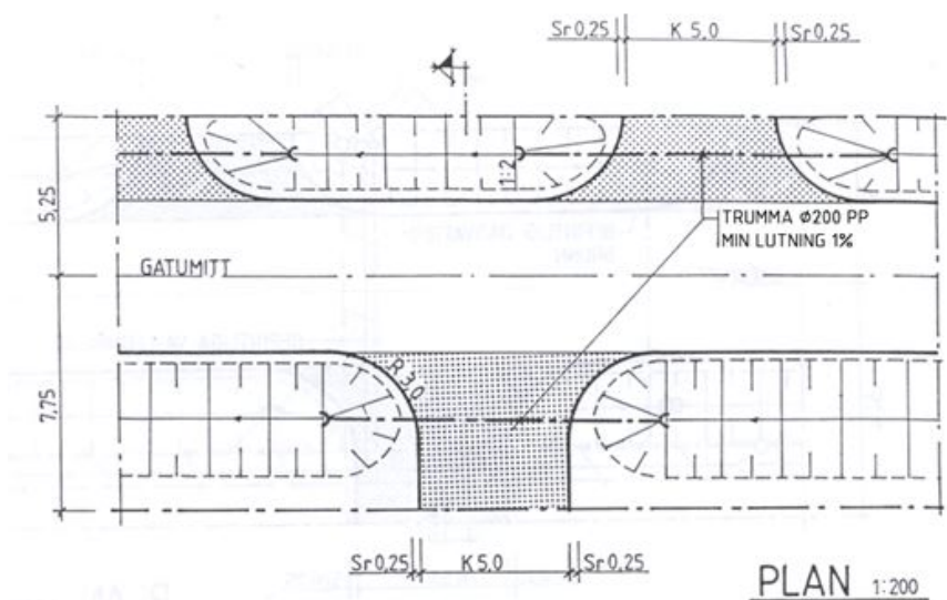
Bild 2 Typsektion vägtrumma
